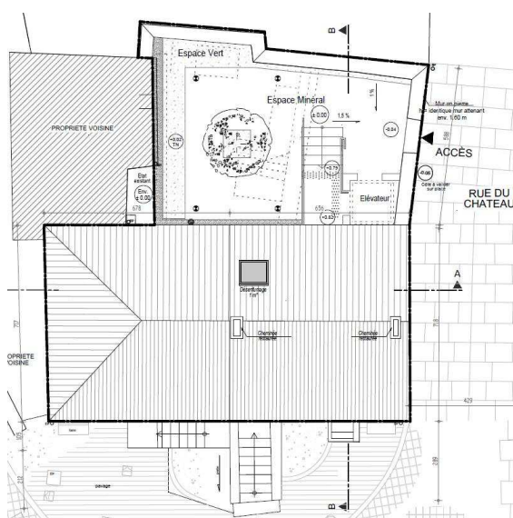
Plan masse
